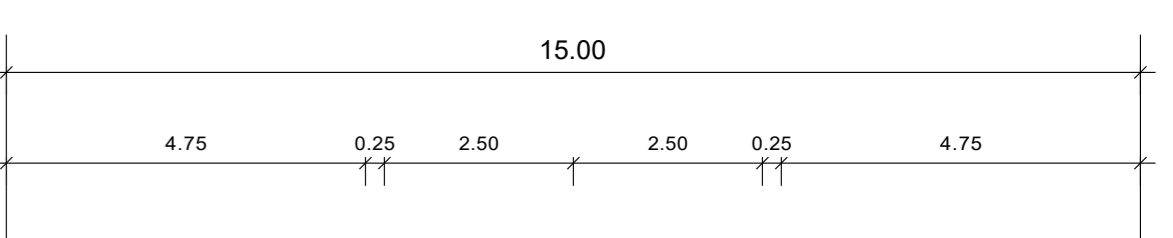
TYYPPIPOIKKILEIKKAUS JYRKÄNPARTAANTIE 1:100
