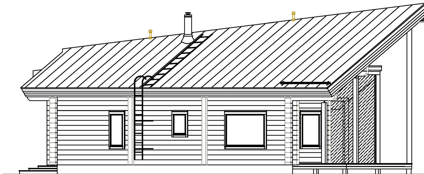
JULKISIVU LUOTEESEEN
