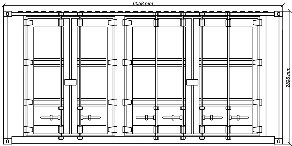
JULKISIVU POHJOISEEN
