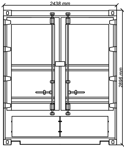
JULKISIVU ITÄÄN
