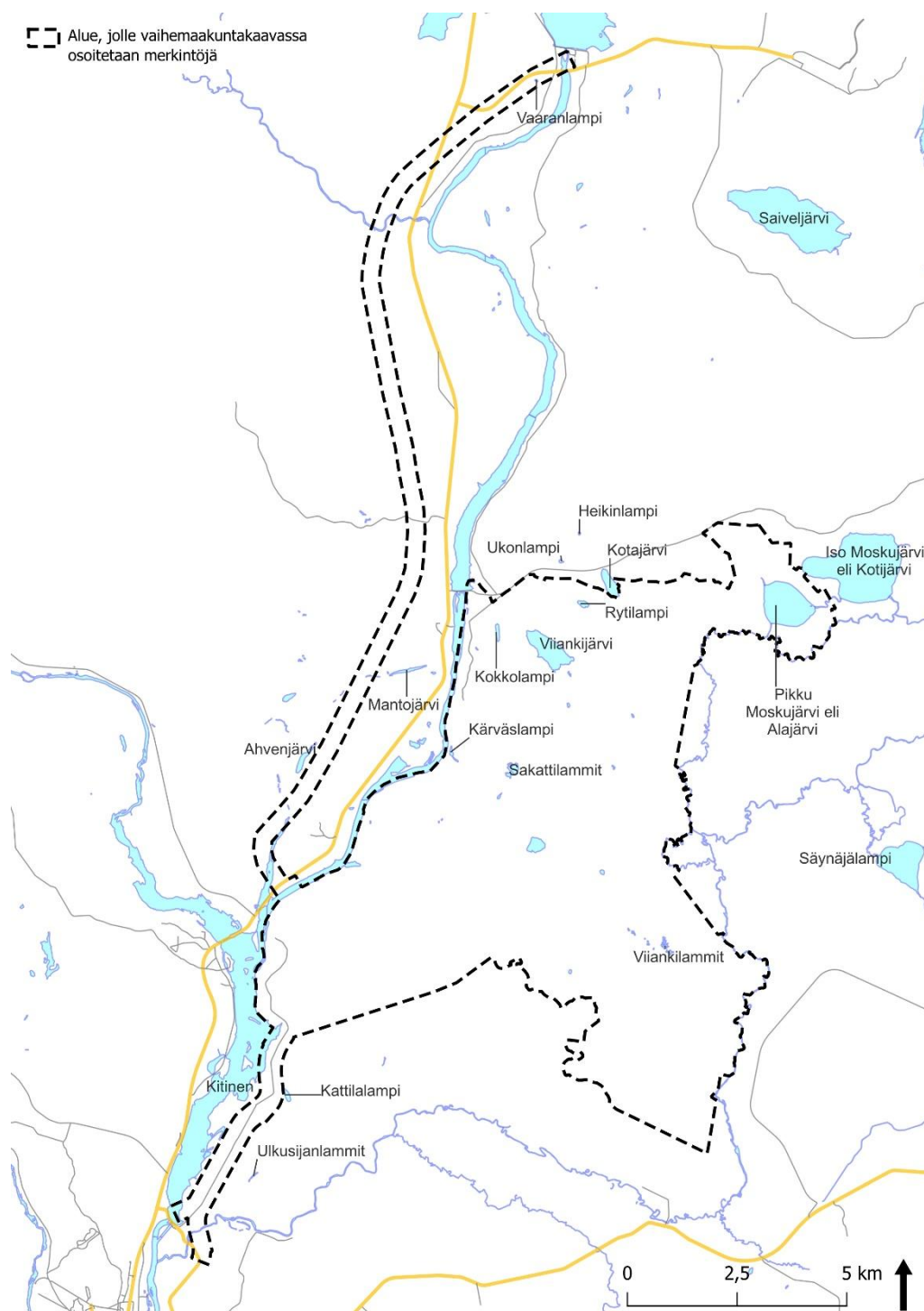
Kuva 8. Vaihemaakuntakaavan suunnittelualueella ja sen läheisyydessä sijaitsevat vesistöt.
