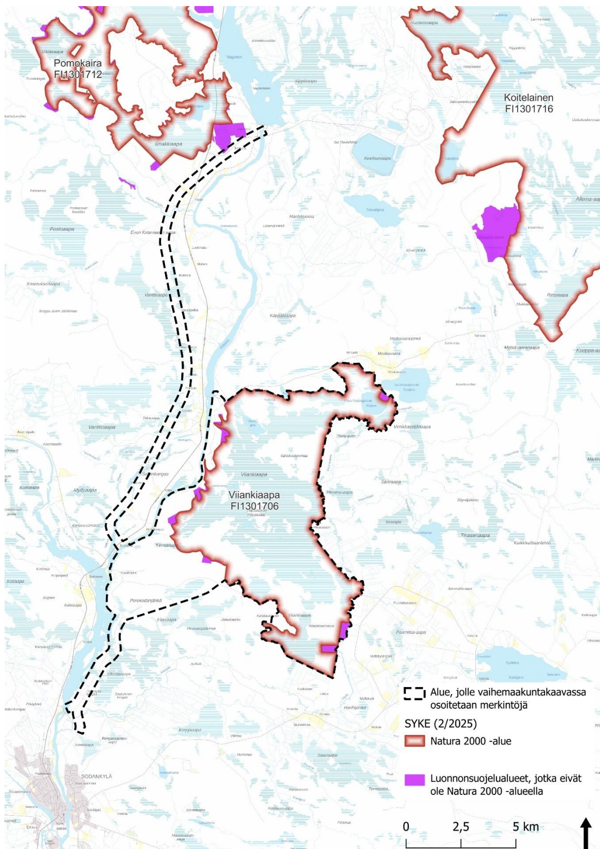
Kuva 13. Natura 2000 -alueet ja luonnonsuojelualueet (valtion omistamat ja yksityisten mailla olevat) niiltä osin, jotka eivät sijaitse Natura 2000 -alueella.
