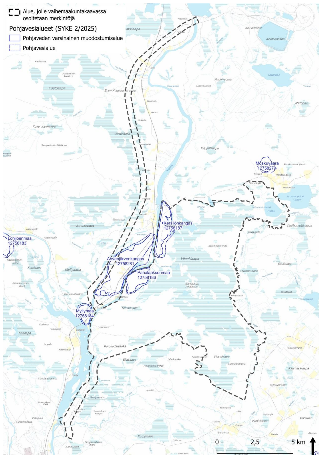
Kuva 10. Vaihemaakuntakaavan suunnittelualueella ja sen läheisyydessä sijaitsevat pohjavesialueet.
