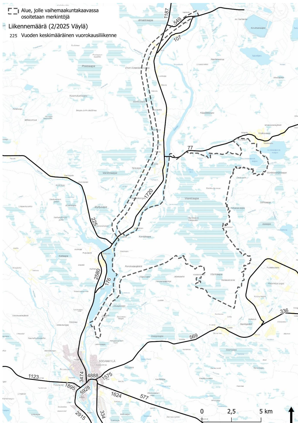
Kuva 16. Keskimääräiset vuorokausiliikennemäärät suunnittelalueen läheisyydessä sijaitsevilla teillä 2025 (Väylävirasto 2025)
