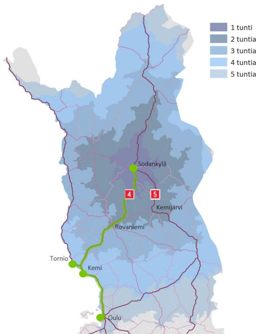
Kuva 23. Raskaan liikenteen arvioidut ajo-ajat Sakatin kaivosalueelta mm. Perämeren satamiin (Sitowise 2024).
