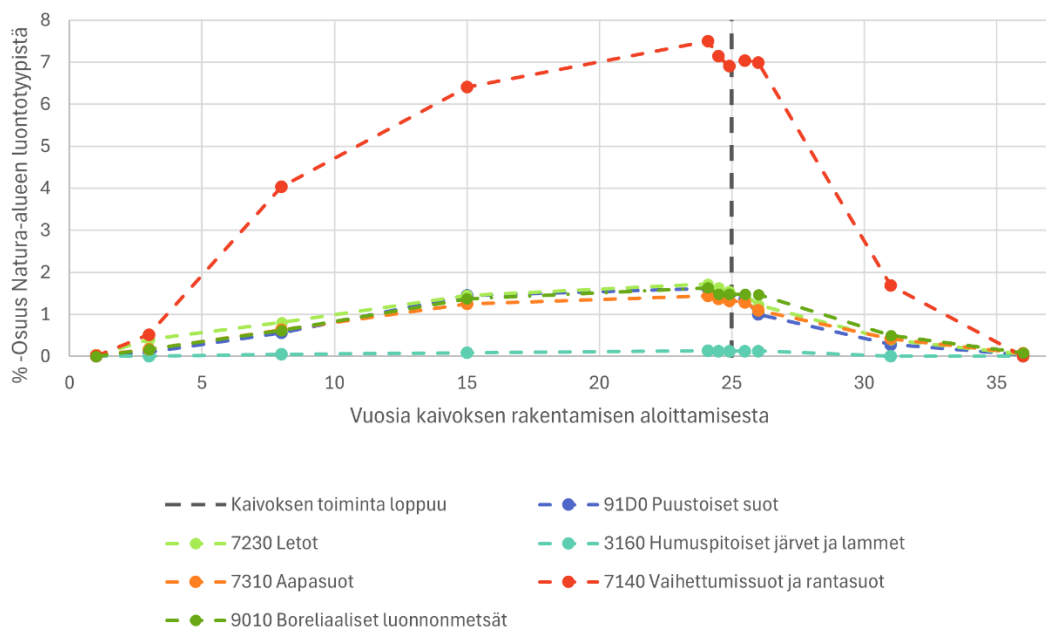
Kuva 21. Vesitaloudellisten vaikutusten vaikutuspiiriin jäävien Viiankiaavan Natura-alueen suojeluperusteena olevien luontotyyppien pinta-alojen kehitys hankkeen elinkaaren aikana, kun toteutetaan Natura-arvioinnissa esitetyt lieventävät toimenpiteet. WSP 2025
