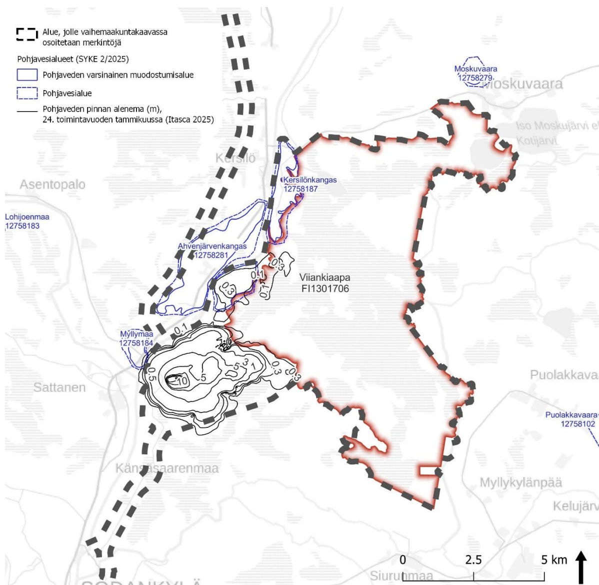
Kuva 18. Mallinnettu pohjaveden pinnan alenema kaivostoiminnan lopussa toimintavuonna 24 65 % tiivistysskenaariossa (ilman NE satelliittisiintymää), pohjavesialueet, ja Natura-alueen raja. (Pohjaveden alenemäkäyrät: Itasca 2025).
