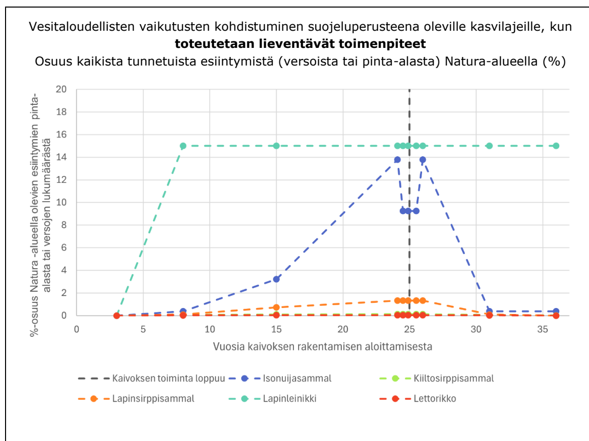
Kuva 22. Vesitaloudellisten vaikutusten kohdentuminen Viiankiaavan suojeluperusteiseen kasvilajistoon, kun hankkeessa toteutetaan Natura-arvioinnissa esitetyt lieventämistoimet.
