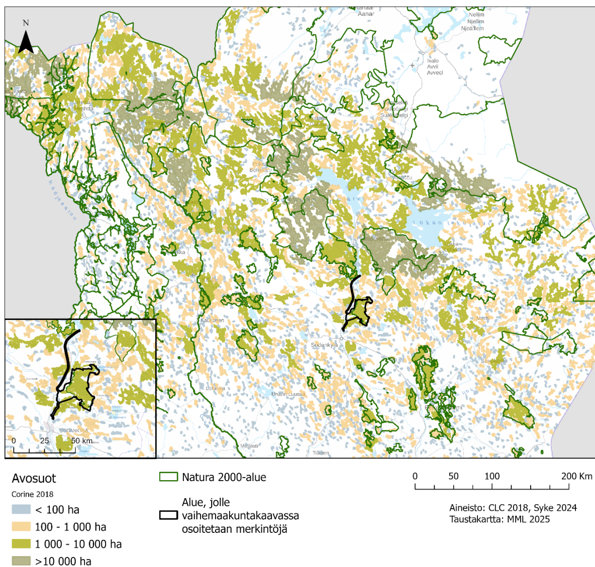
Kuva 11. Sakatin vaihemaakuntakaavassa osoitettavien merkintöjen sijainti Lapin avosoihin ja Natura-alueisiin nähden.
