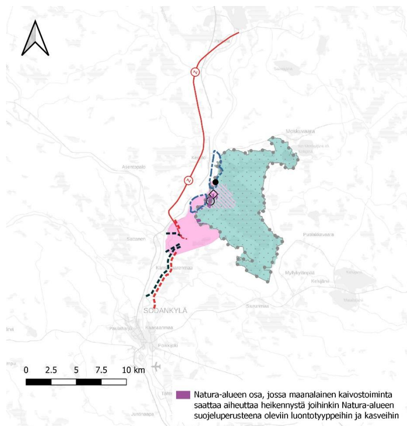
Kuva 20. Vaihemaakuntakaavan merkintöjen päällä on esitetty Natura-alueen osa, jossa maanalainen kaivostointa saattaa aiheuttaa heikennystä joihinkin Natura-alueen suojeluperusteena oleviin luontotyyppisiin ja kasveihin.
