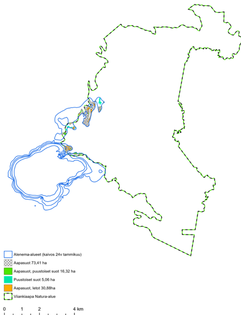
Kuva 19. Viiankiaavan Natura-alueen osat, jossa maanalainen kaivostoiminta saattaa aiheuttaa heikennystä joihinkin Natura-alueen suojeluperusteena oleviin luontotyyppeihin ja kasveihin. Kuvassa on esitetty pohjaveden alenema-alueet myös Natura-alueen ulkopuolella.
